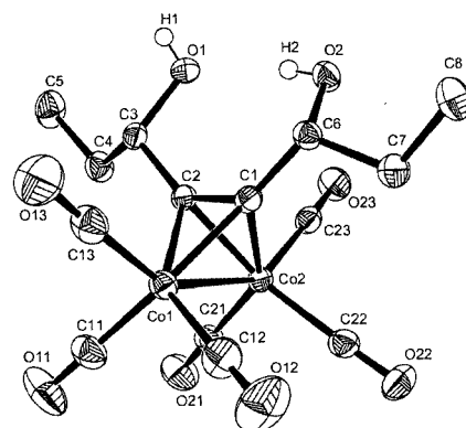
meso - 9b
