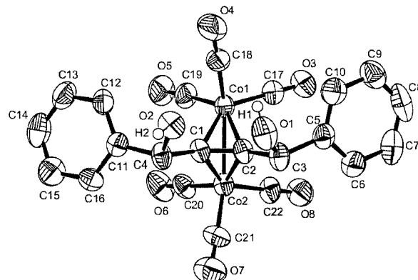
meso - 9d
